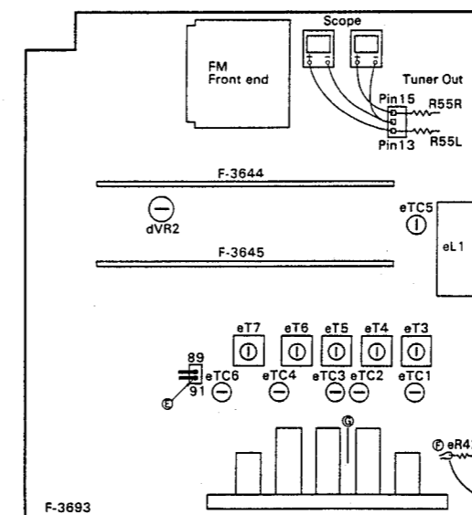
Fig. 3-7 <CP-R7>
