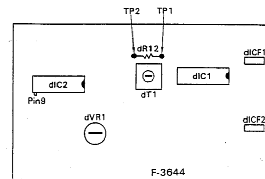
Fig. 3-5 <CP-R7/CP-R5>
